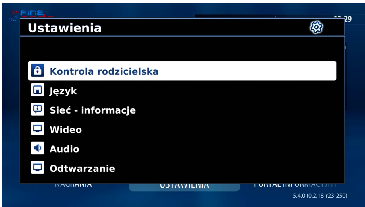
Ustawienia dekodera
